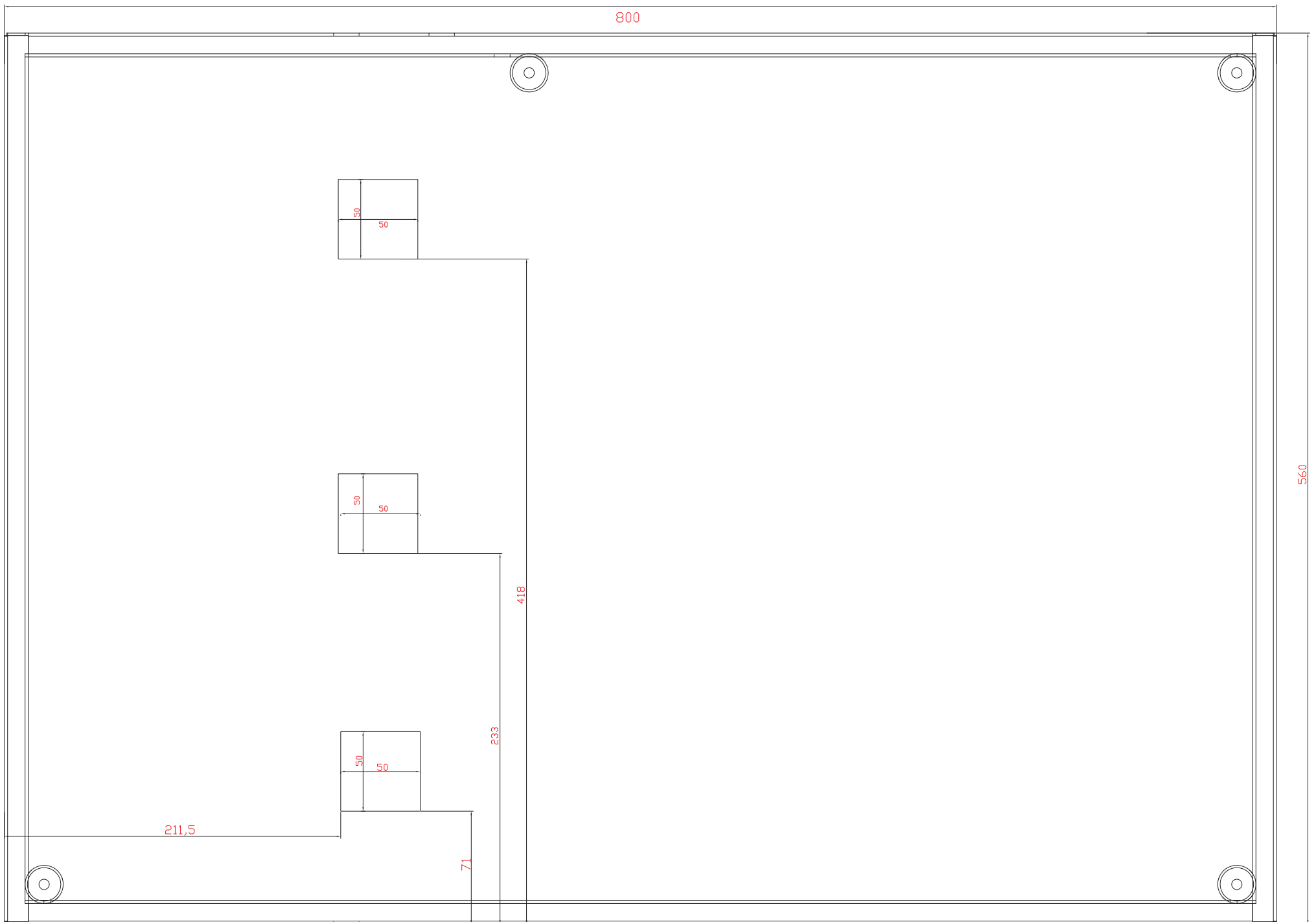
KD7v2-80 Ansicht Befestigungen und Kabeleinführungen
